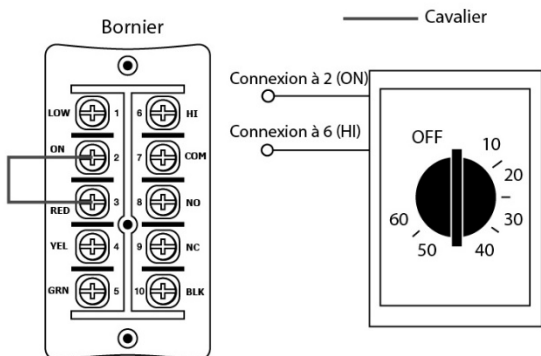
Connexions de contacts secs avec bornier de type A
