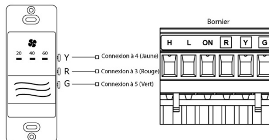
Minuterie DET01 avec bornier de type B
