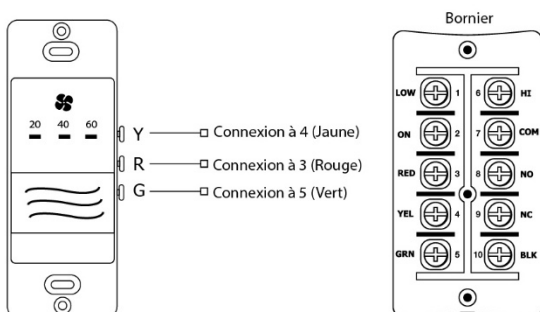
Minuterie DET01 avec bornier de type A
