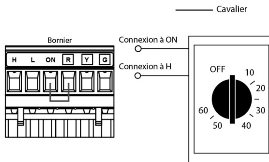
Connexions de contacts secs avec bornier de type B
